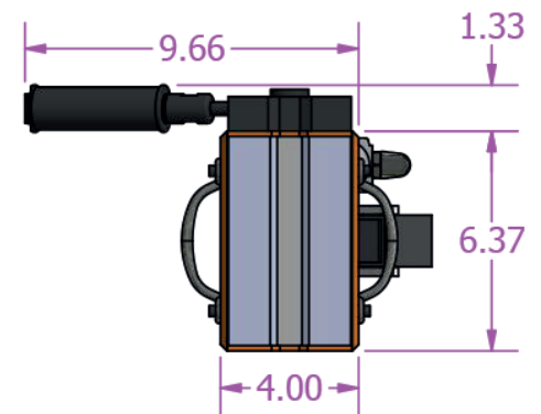
VIEW A-A
